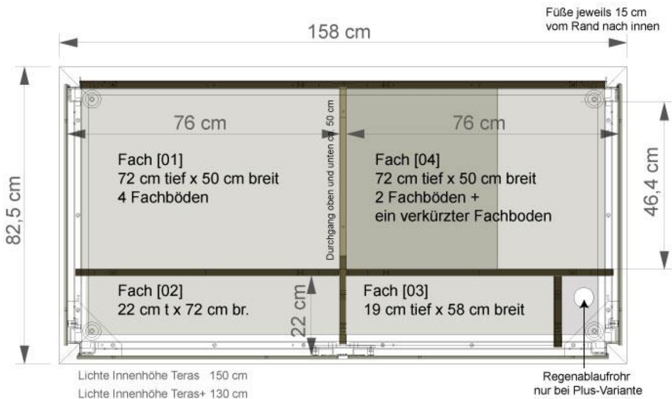
Grundriss Garten[Q]Teras-3 in der Ausführung mit Zugriff von drei Seiten
